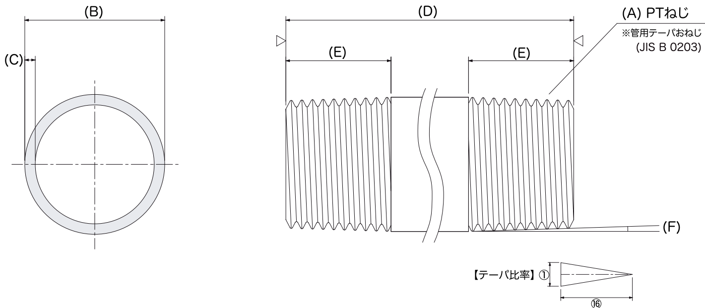
【ねじ詳細図】
